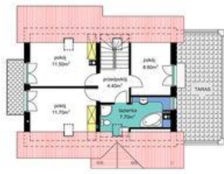
PODDASZE Pu-43.90m 2 , p.podł.-58.50m 2
