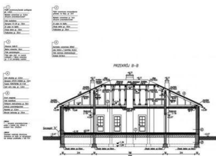
Przekrój B-B
