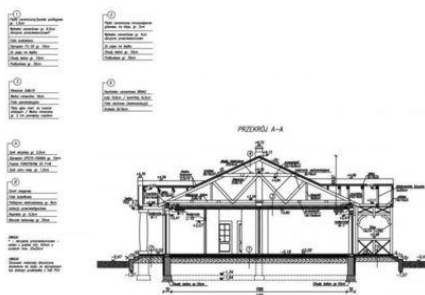
Przekrój A-A
