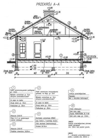
Przekrój A-A
