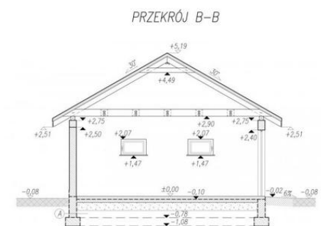
Przekrój B-B
