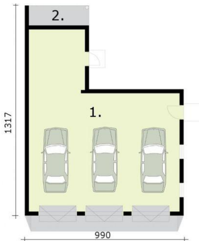
Rzut przyziemia 1. Garaż 83.7m 2 2. Skład na drewno 4.63m 2
