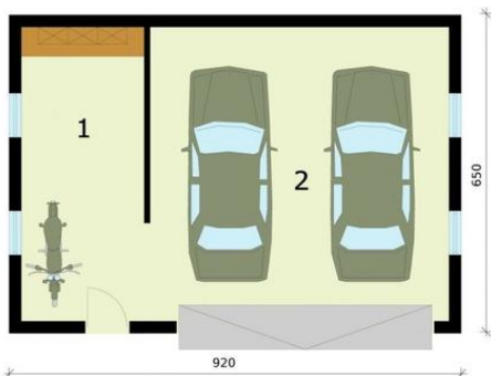
Rzut przyziemia 1 Pomieszczenie gospodarcze 15.65m 2 2 Garaż 36.84m 2
