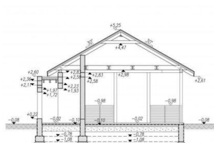
Przekrój B-B
