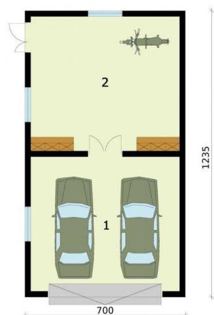
Rzut przyziemia 1. Garaż 37.7m 2 2. Pom. Gospodarcze 37.7m 2
