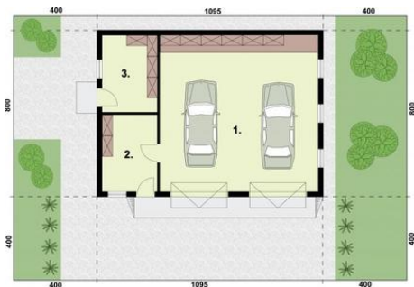
Rzut przyziemia 1. Garaż 57.45m 2 2. Pomieszczenie gosp. 9.85m 2 3. Pomieszczenie gosp. 9.85m 2
