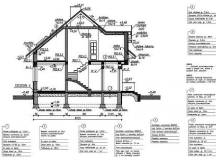
Przekrój A-A
