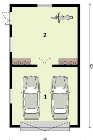
Rzut przyziemia 1. Garaż 37.33m 2 2. Pom. gospodarcze 37.33m 2
