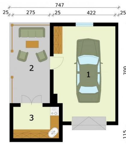
Rzut przyziemia 1. Garaż 26.33m 2 2. Weranda 14.14m 2 3. Pom. gospodarcze 6.55m 2
