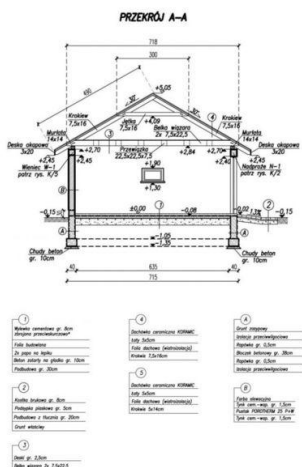
Przekroj A-A
