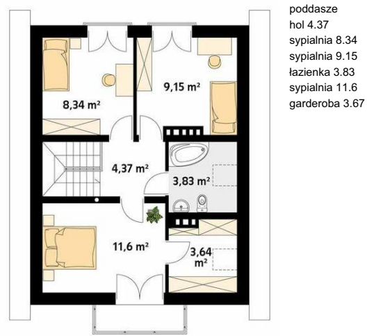
Poddasze
