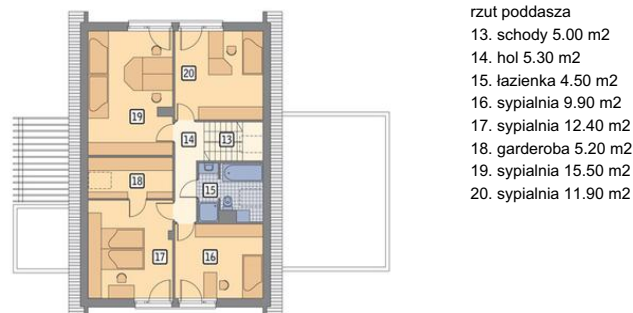
Poddasze
