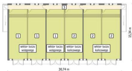
rzut przyziemia
