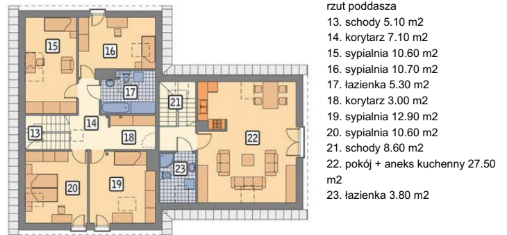
Poddasze
