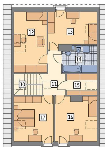
Poddasze
