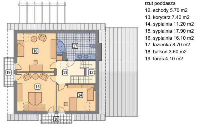
Poddasze
