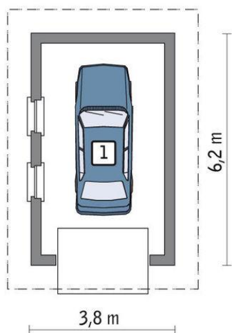
rzut parteru 1. garaż 19.70 m 2
