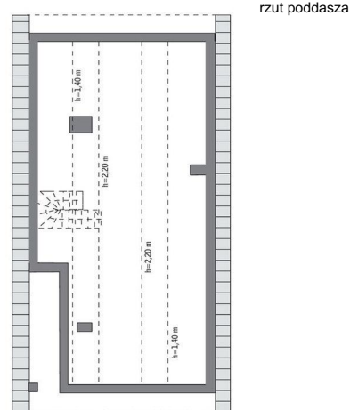
Poddasze
