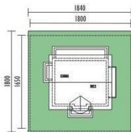
Minimalne wymiary działki 1:500 (wymiar mniejszy realizowy przy zamianie tarasów na ziemię)
