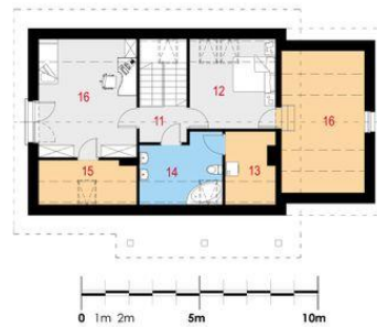
Poddasze
