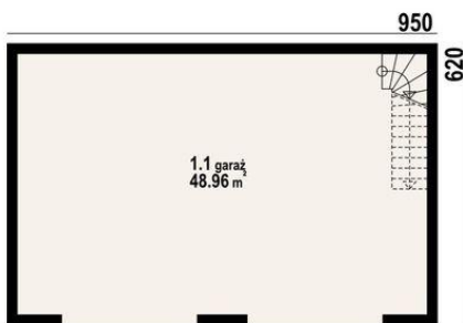
1.1 - garaż - 48.96 m 2
