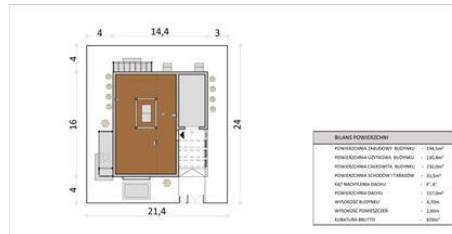
Projekt domu AJR 23 - rzut parteru
